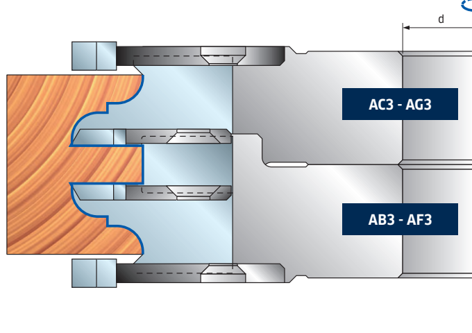
Example of scribe Esempio di controprofilo
